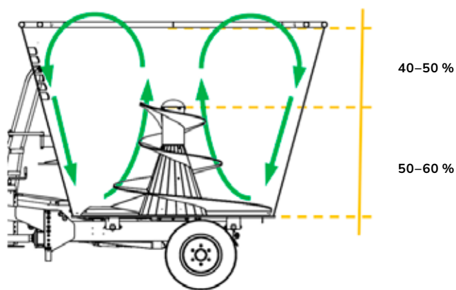
Högt volymutnyttjande. Perfekt samspel mellan blandarskruv och blandarkar.
