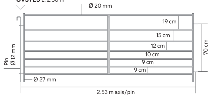
OV3725 L. 2.50 m
